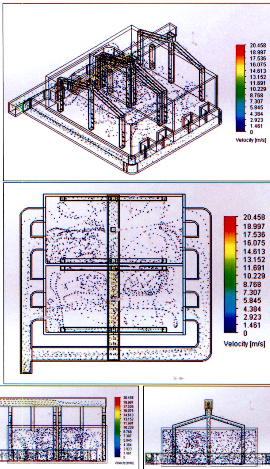
ภาพที่ 26 ผลการจำลองการไหลของไอเสียของต้นแบบห้องอบแห้งแบบที่ 3
