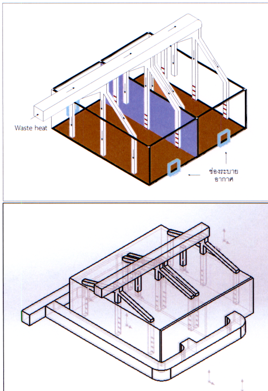
ภาพที่ 23 แบบแปลนต้นแบบห้องอบแห้งแบบที่ 2
