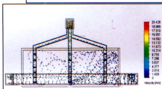
ภาพที่ 32 ผลการจำลองการไหลของไอเสียของต้นแบบห้องอบแห้งแบบที่ 6
