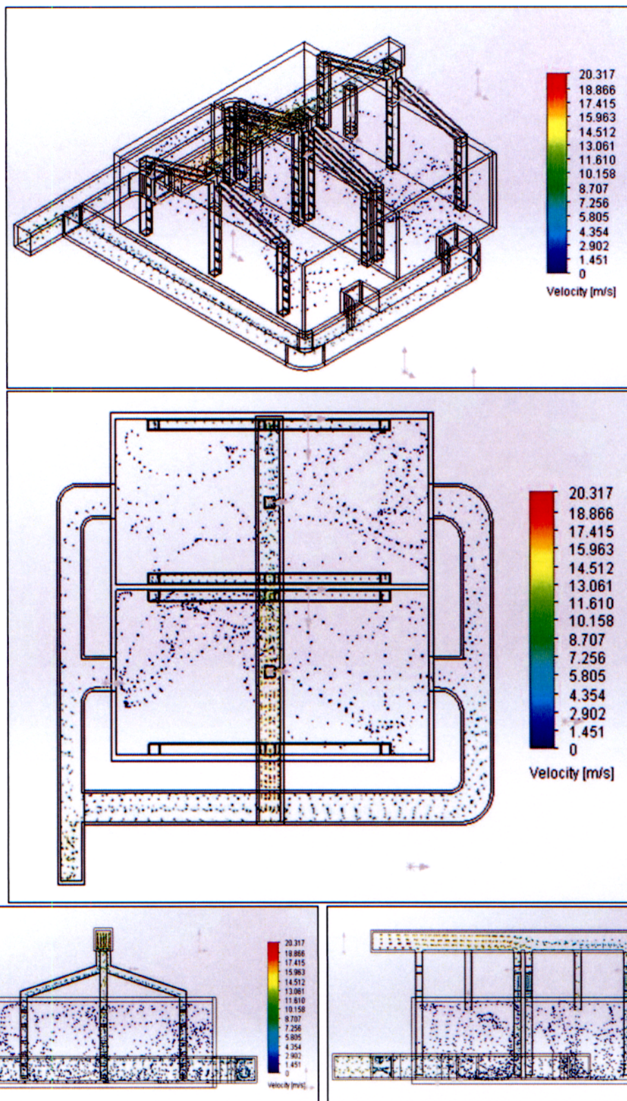
ภาพที่ 30 ผลการจำลองการไหลของไอเสียของต้นแบบห้องอบแห้งแบบที่ 5
