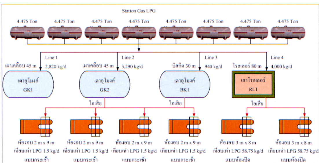
ภาพที่ 9 แผนภาพกระบวนการใช้แก๊ส LPG ของบริษัท กาสะลอง เซรามิกส์ จำกัด (Zone 1)
