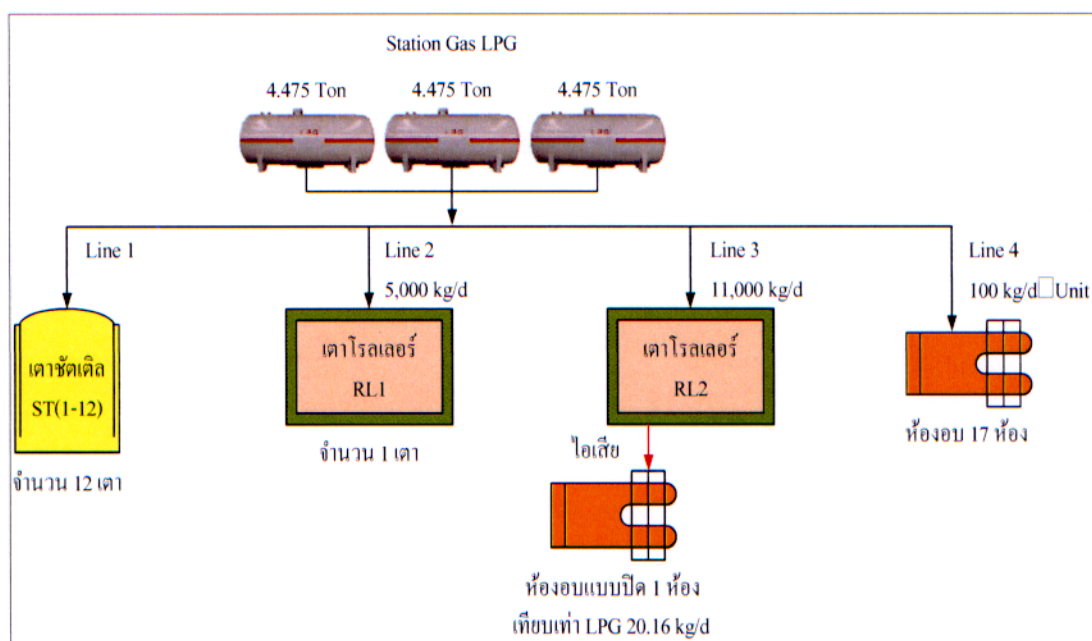
ภาพที่ 6 แผนภาพกระบวนการใช้แก๊ส LPG ของบริษัท อินทราเซรามิค จำกัด
