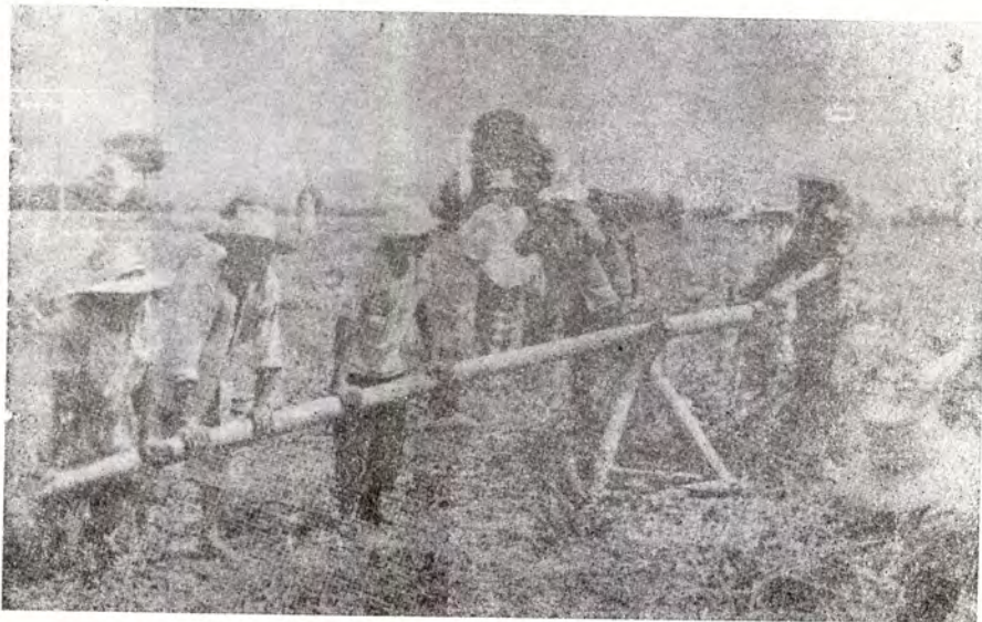
สามขา (คานงัด) ที่ใช้ผูกเหง้าไถ่คืนขึ้น สามขา ๑ ตัว จะใช้คนงาน ๕ คน
